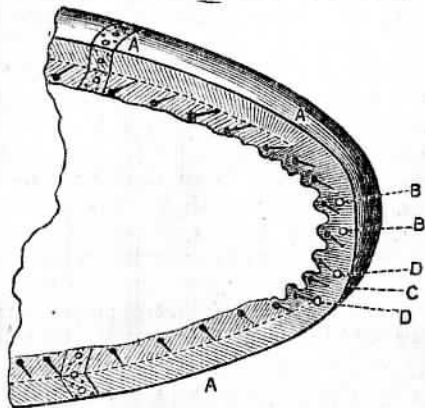
Fig. 87.—Lasting the Toe.
