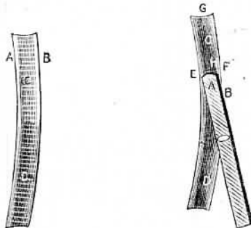
Fig. 144.—Peening Edge of Sole. Fig. 145.—Rasping Edge of Sole.
