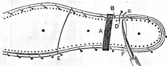
Fig. 90.—Sewing the Welt.
