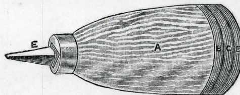
Fig. 4.—Home-made Awl.
